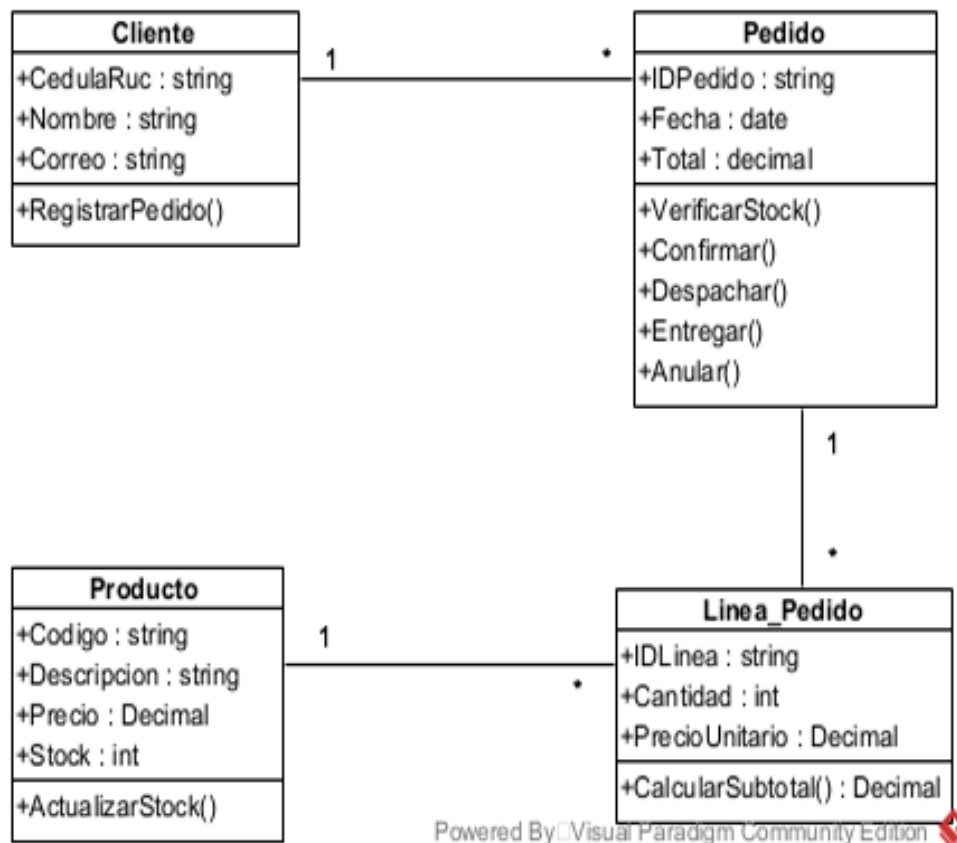
Figura 1: Diagrama de Clases UML — Dominio del Sistema de Pedidos.
